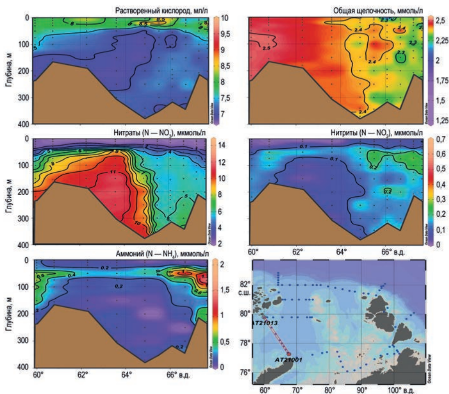
Рис. 3.3.3. Вертикальное распределение содержания растворенного кислорода (мл/л), общей щелочности (ммоль/л), нитратов ( N - NO_3 , мкмоль/л), нитритов ( N - NO_2 , мкмоль/л), аммонийного азота ( N - NH_4 , мкмоль/л) и схема расположения разреза.
