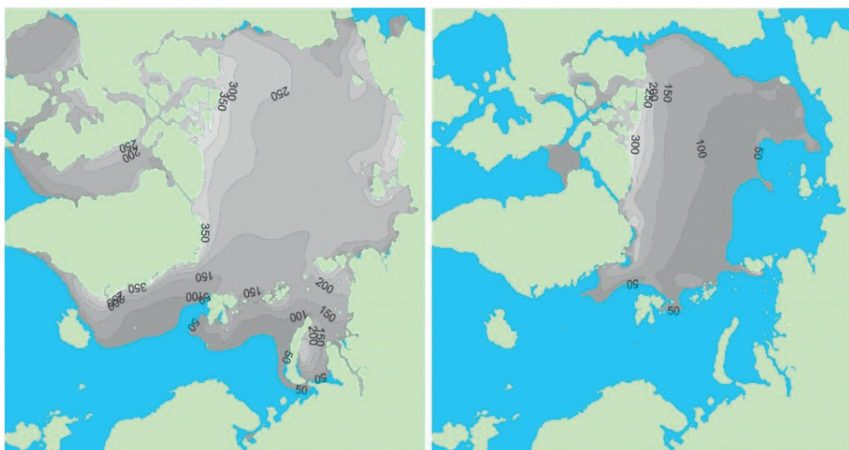
Рис. 2.3.10. Распределение средней толщины льда (с учетом торосов) в СЛО по результатам расчетов на 1 мая (слева) и 1 октября (справа) 2021 г.
