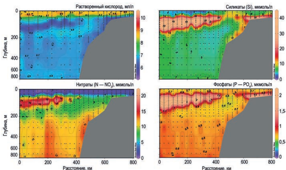
Рис. 3.3.5. Вертикальное распределение растворенного кислорода, мл/л, силикатов (Si, мкмоль/л), нитратного азота (N — NO 3 , мкмоль/л) и фосфатов (P — PO 4 , мкмоль/л) на разрезе через центральную часть шельфа и континентальный склон Восточно-Сибирского моря.
