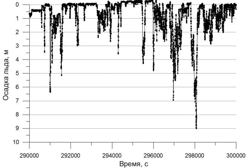
Рис. 4. Фрагмент данных сканирования нижней поверхности ледяного покрова Fig. 4. Fragment of data of ice cover lower surface scanning
