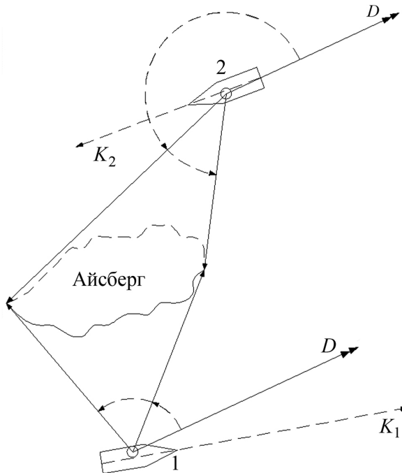
Рис. 7. Схема наблюдения за айсбергом с помощью тахеометра Fig. 7. Scheme of the observation on the iceberg using a tacheometer
