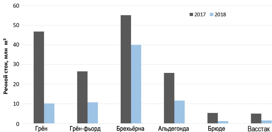
Рис. 3. Объемы общего и ледникового стоков (млн м 3 ) по данным 2017 и 2018 гг. на реках Грён-фьорда
